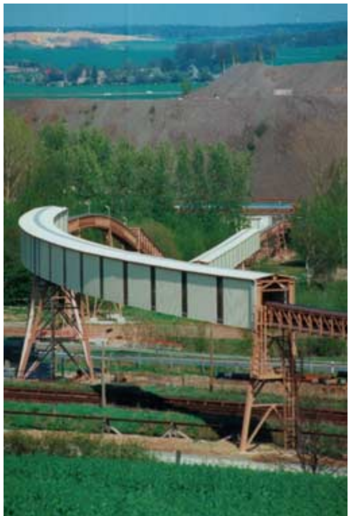
Pipe-Conveyor – Geschlossener kurvengängiger Gurtbandförderer zum Transport von Bergematerial des Standortes Crossen zur Sanierung der Absetzanlage Helmsdorf (Foto: WISMUT GmbH)
